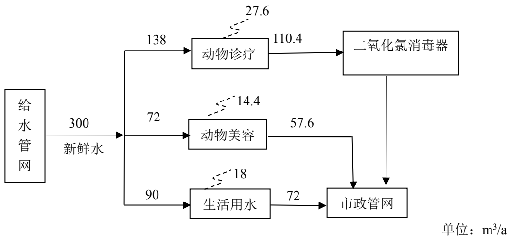
图 1 水平衡图
