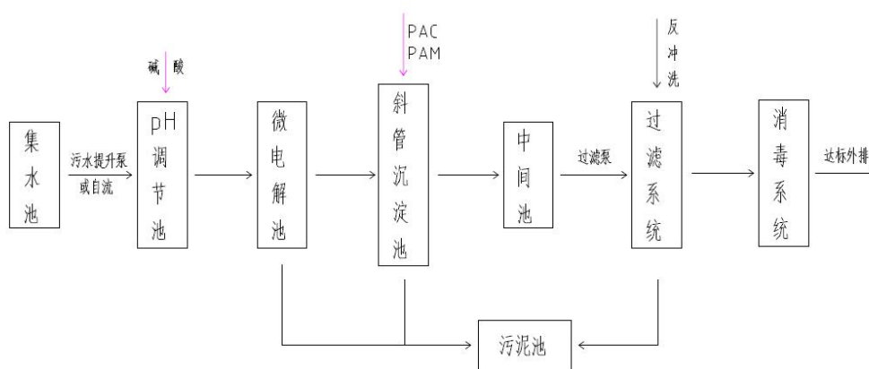
图 5 污水处理工艺流程
