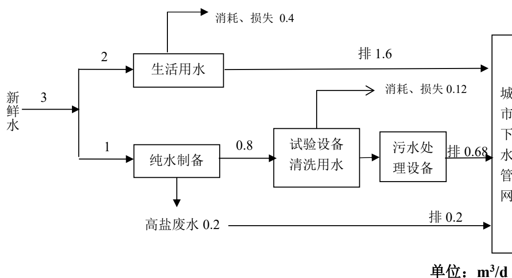
图 1 项目水量平衡图
